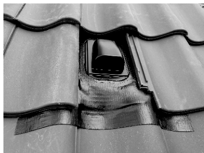
TUSSEN de pannen
